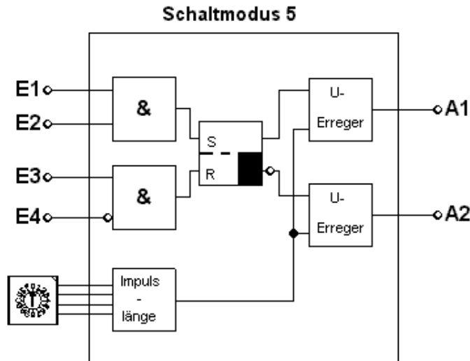
Abbildung 6: Schaltmodus 5
