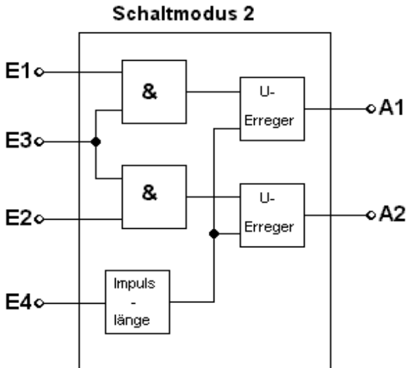
Abbildung 3: Schaltmodus 2
