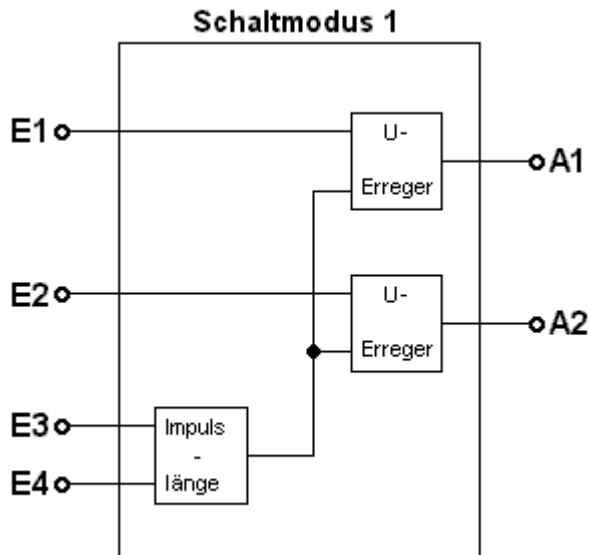
Abbildung 2: Schaltmodus 1
