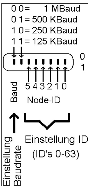
Bild 3: DIP-Switch
