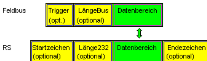
Datenaufbau Universales 232 Protokoll
