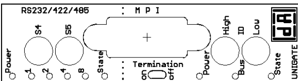
Bild 2: Frontblende: Drehschalter, Leuchtanzeigen und Terminierung MPI
